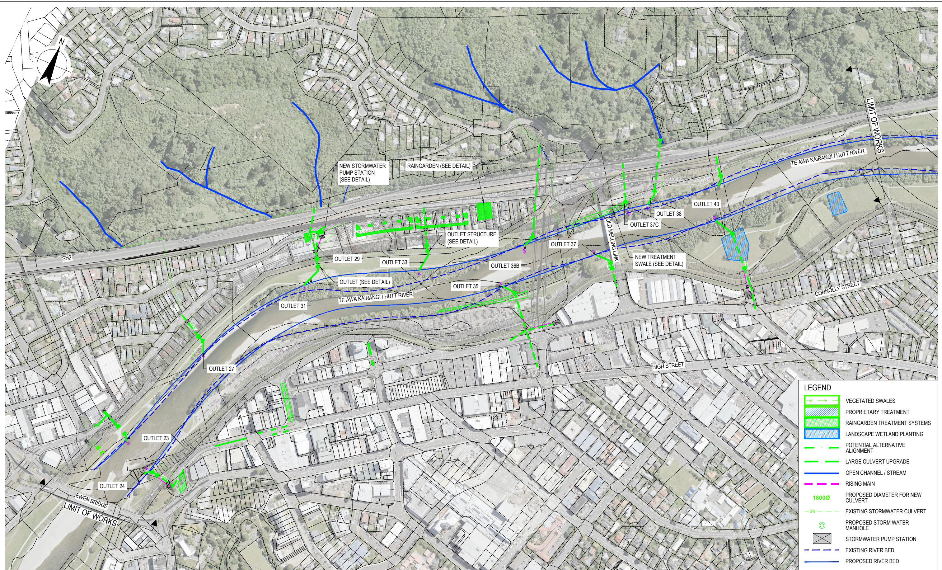
PLAN SCALE 1 : 2500
